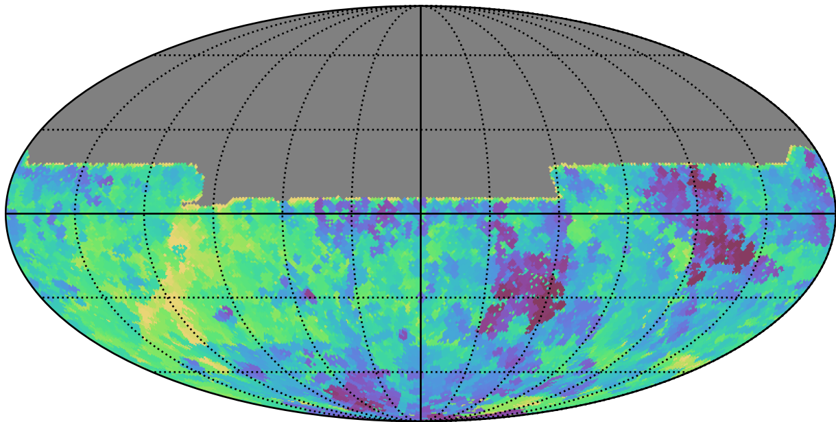
too_100_1v3.4_10yrs All sky y band: Min saturation_mag
