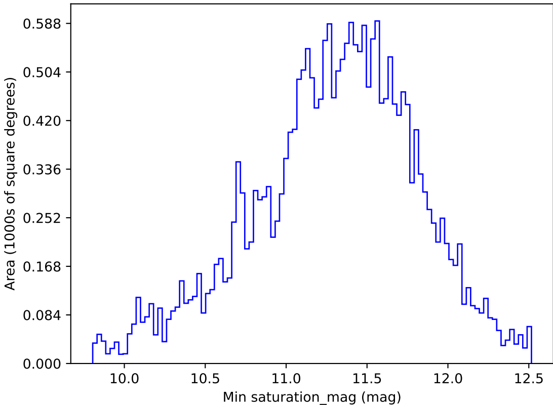
too_100_1v3.4_10yrs All sky y band: Min saturation_mag
