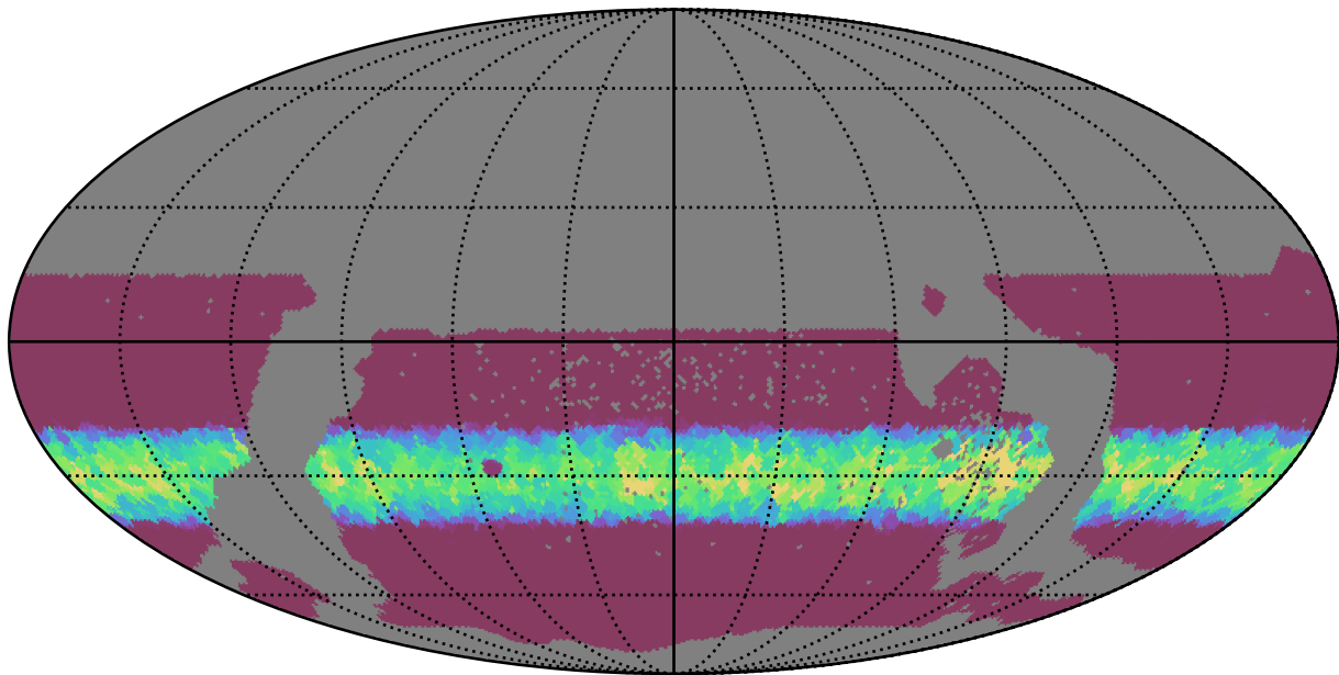
too_100_1v3.4_10yrs WFD y band: Min normairmass
