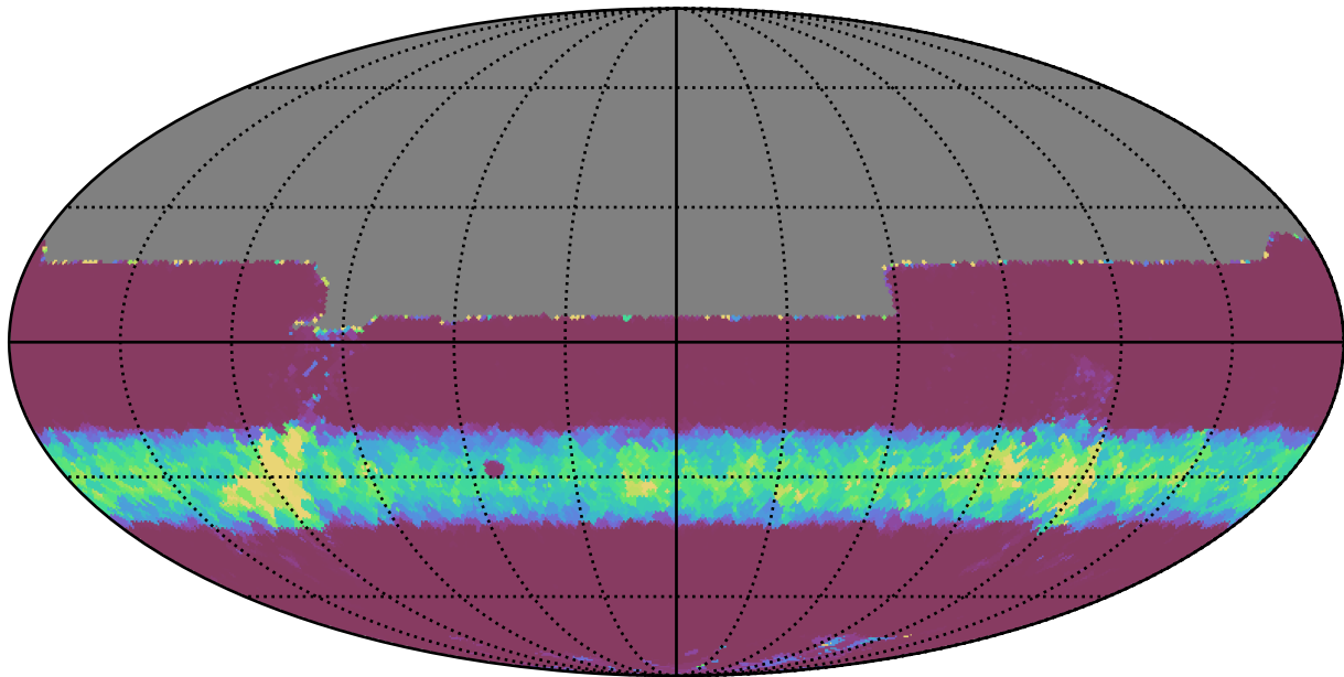
too_100_1v3.4_10yrs All sky y band: Min normairmass
