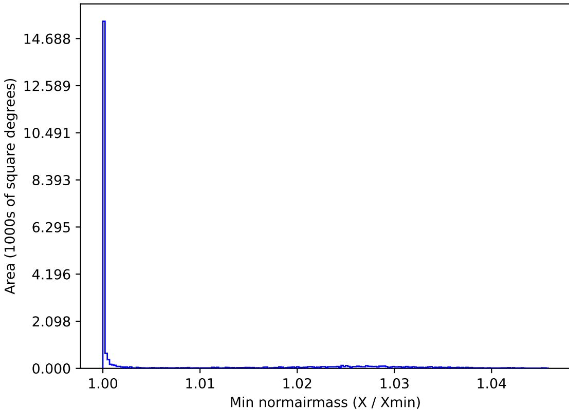
too_100_1v3.4_10yrs All sky y band: Min normairmass
