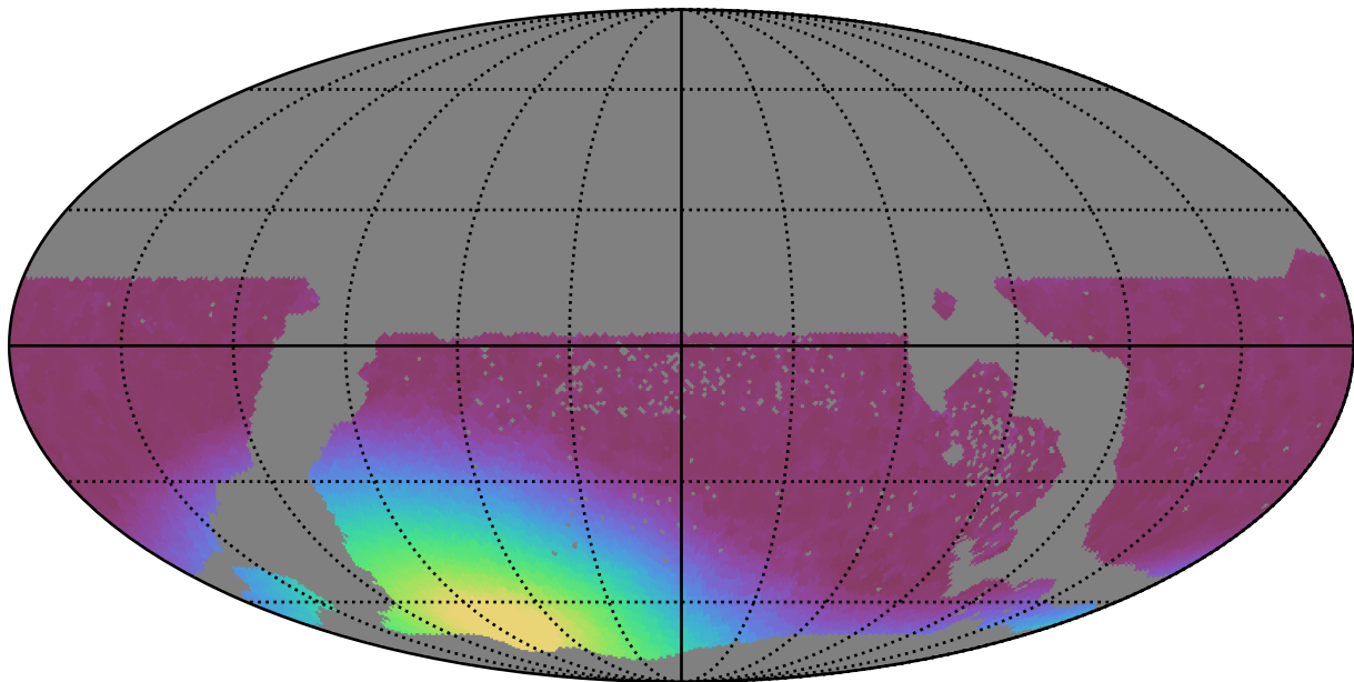
too_100_1v3.4_10yrs WFD y band: Min moonDistance
