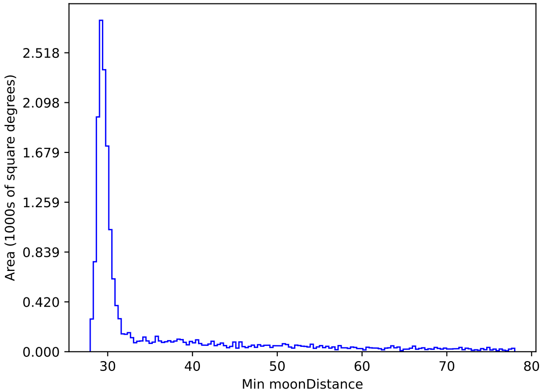
too_100_1v3.4_10yrs WFD y band: Min moonDistance
