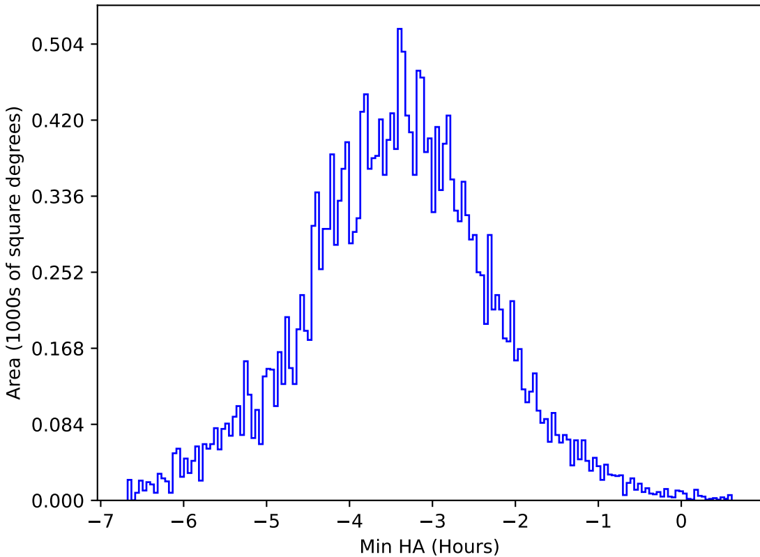
too_100_1v3.4_10yrs All sky y band: Min HA
