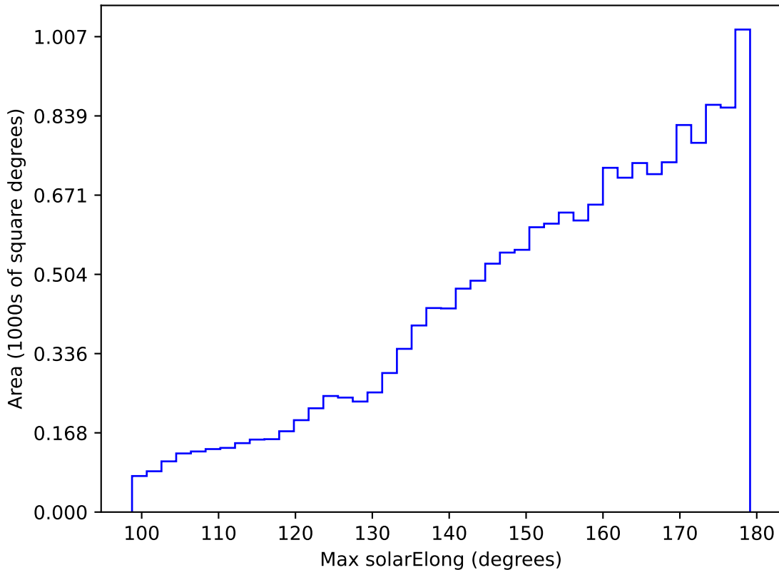
too_100_1v3.4_10yrs WFD y band: Max solarElong
