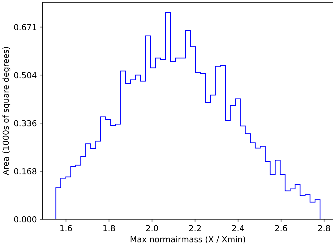
too_100_1v3.4_10yrs WFD y band: Max normairmass
