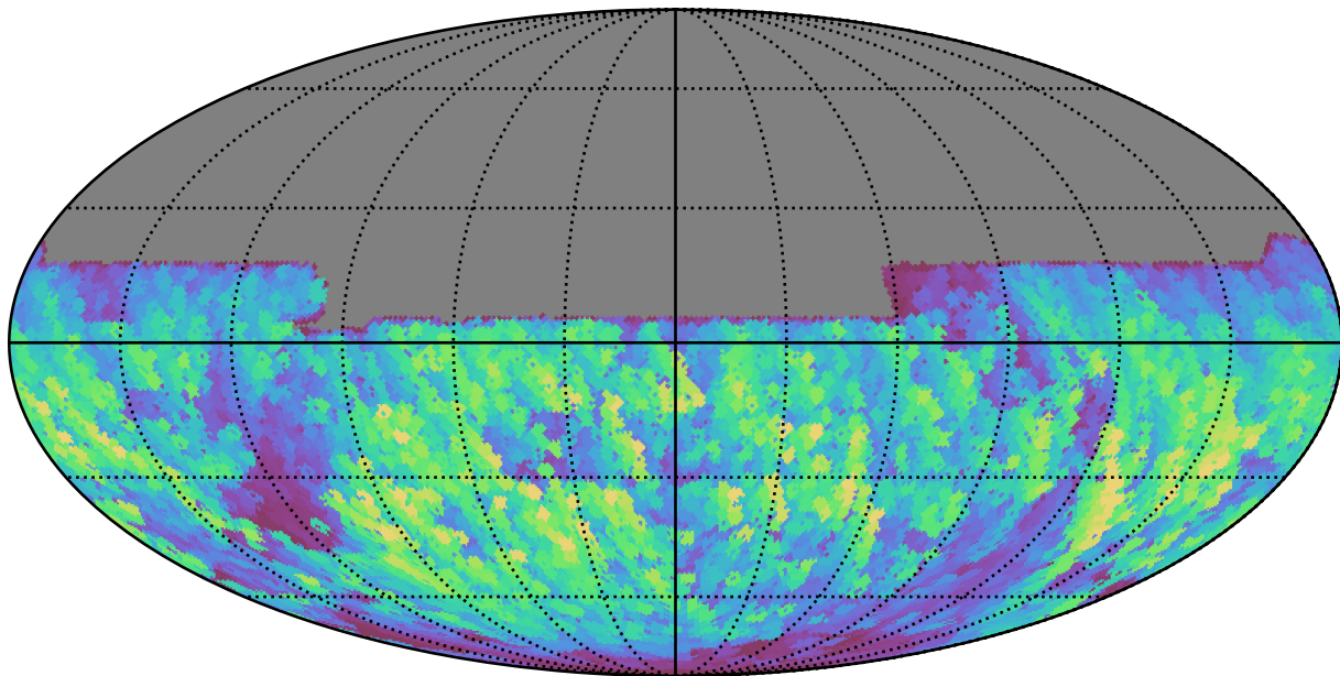
too_100_1v3.4_10yrs All sky y band: Max normairmass
