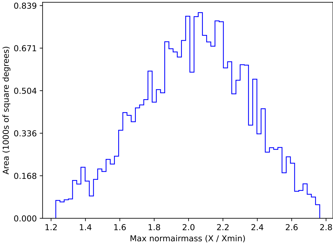
too_100_1v3.4_10yrs All sky y band: Max normairmass
