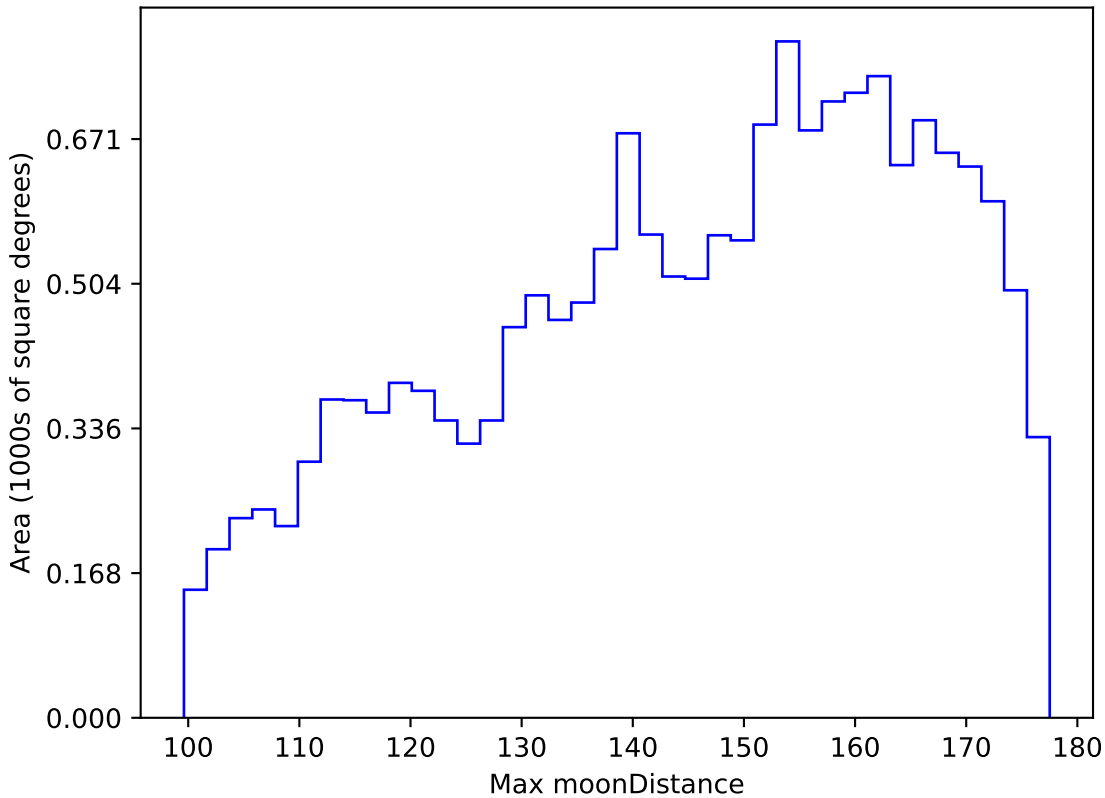
too_100_1v3.4_10yrs WFD y band: Max moonDistance
