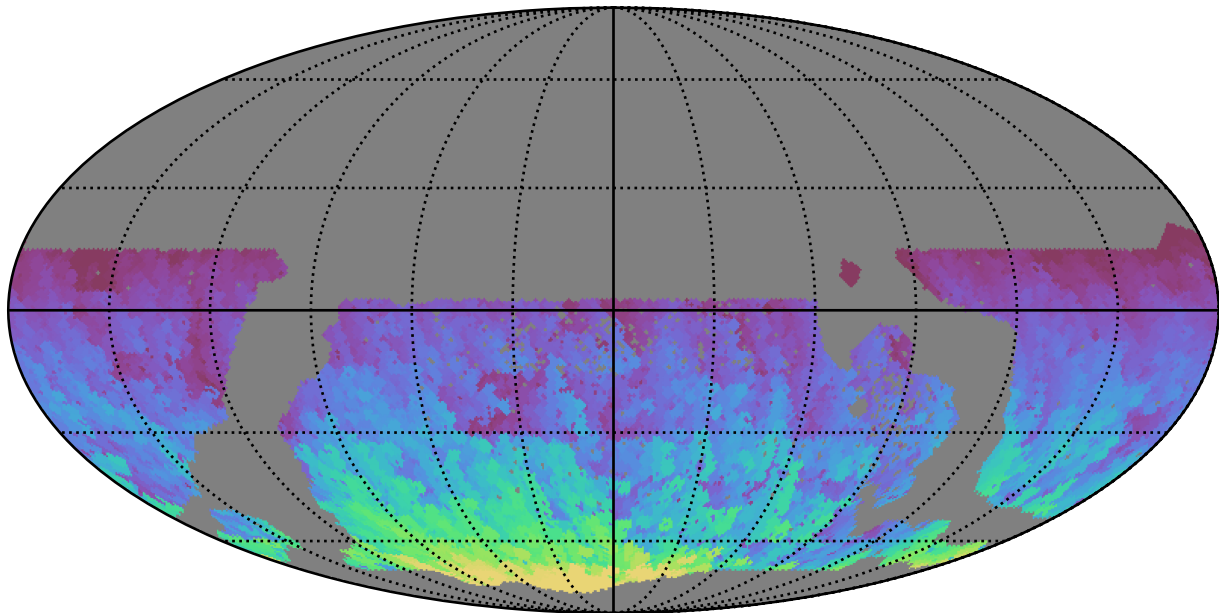
too_100_1v3.4_10yrs WFD y band: Max HA
