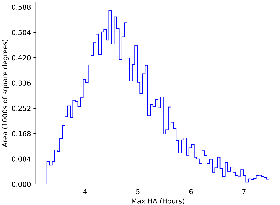
too_100_1v3.4_10yrs WFD y band: Max HA
