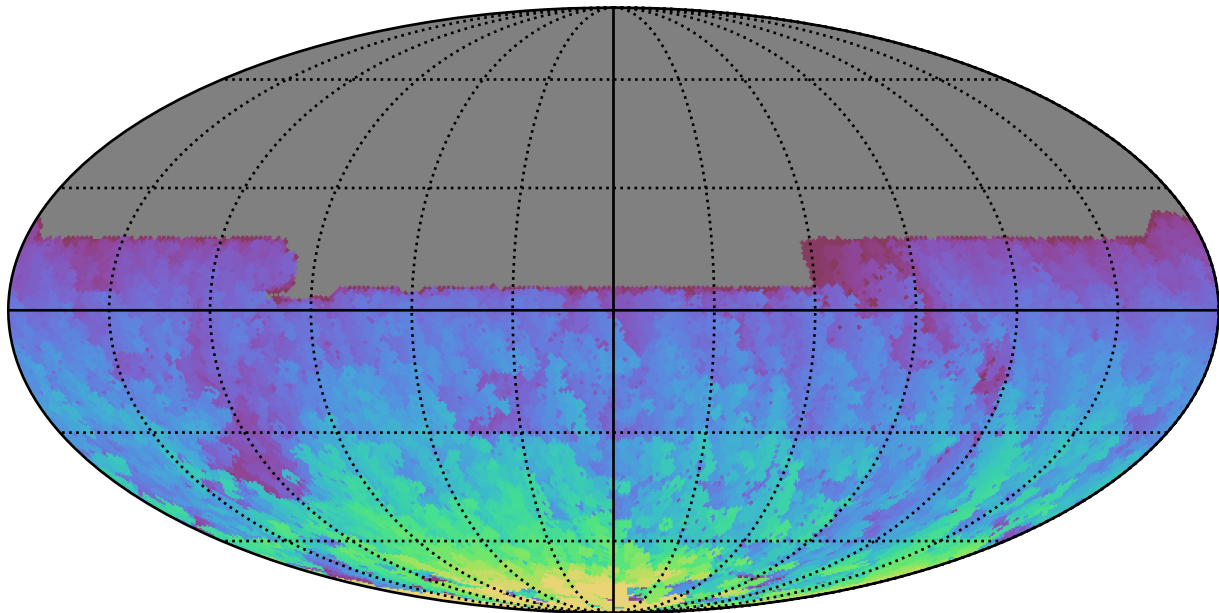
too_100_1v3.4_10yrs All sky y band: Max HA
