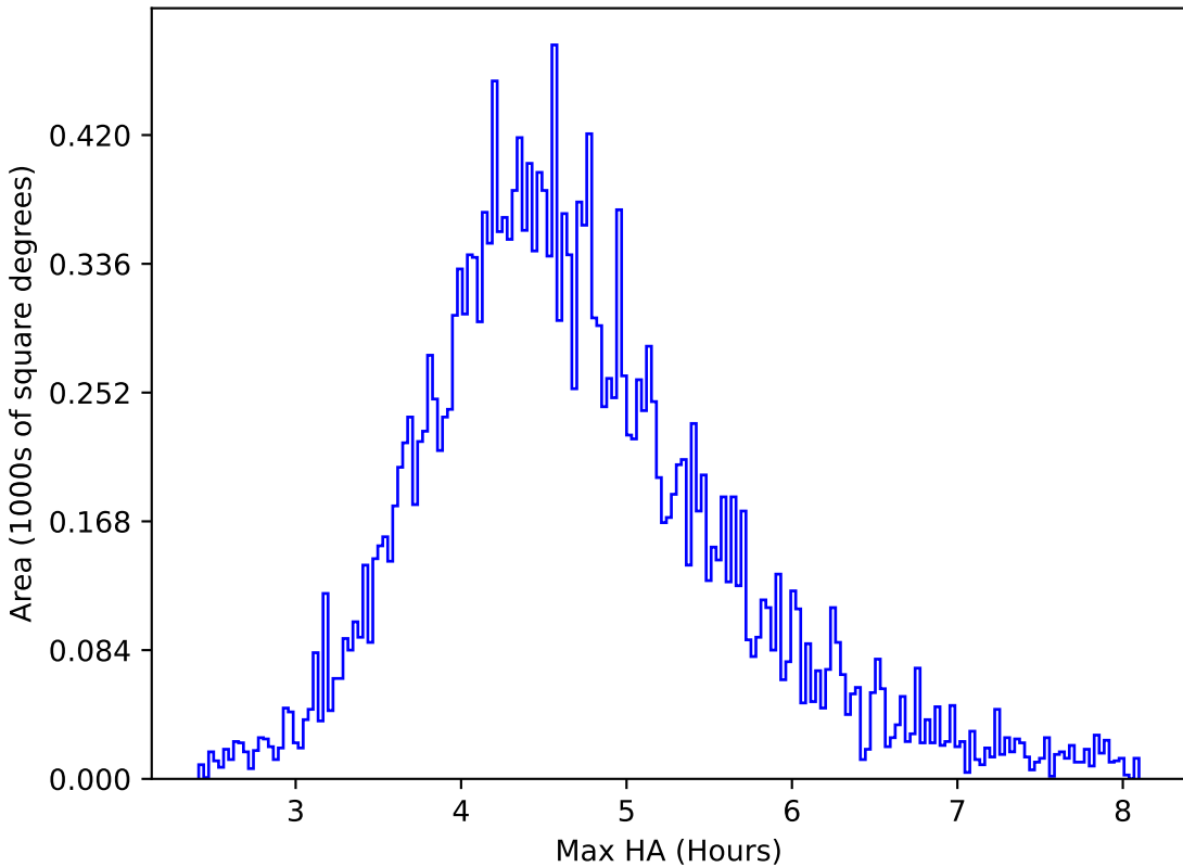
too_100_1v3.4_10yrs All sky y band: Max HA
