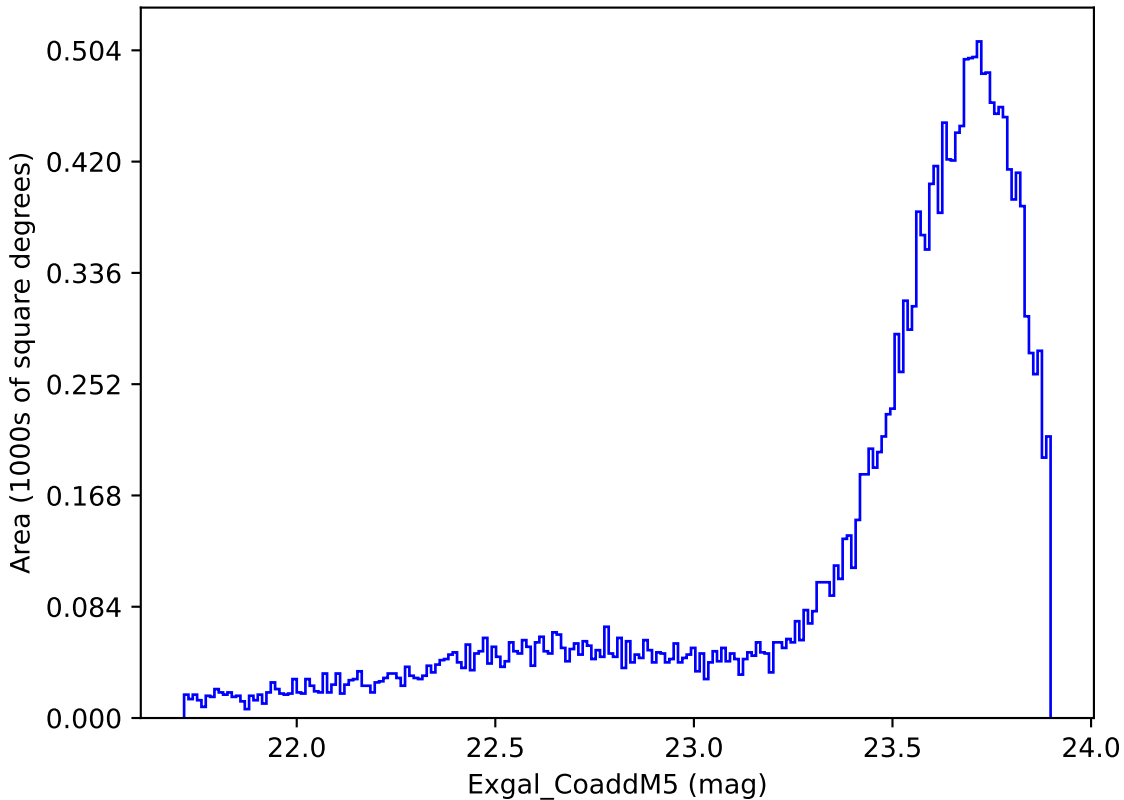
too_100_1v3.4_10yrs Yr 1 y band: Exgal_CoaddM5
