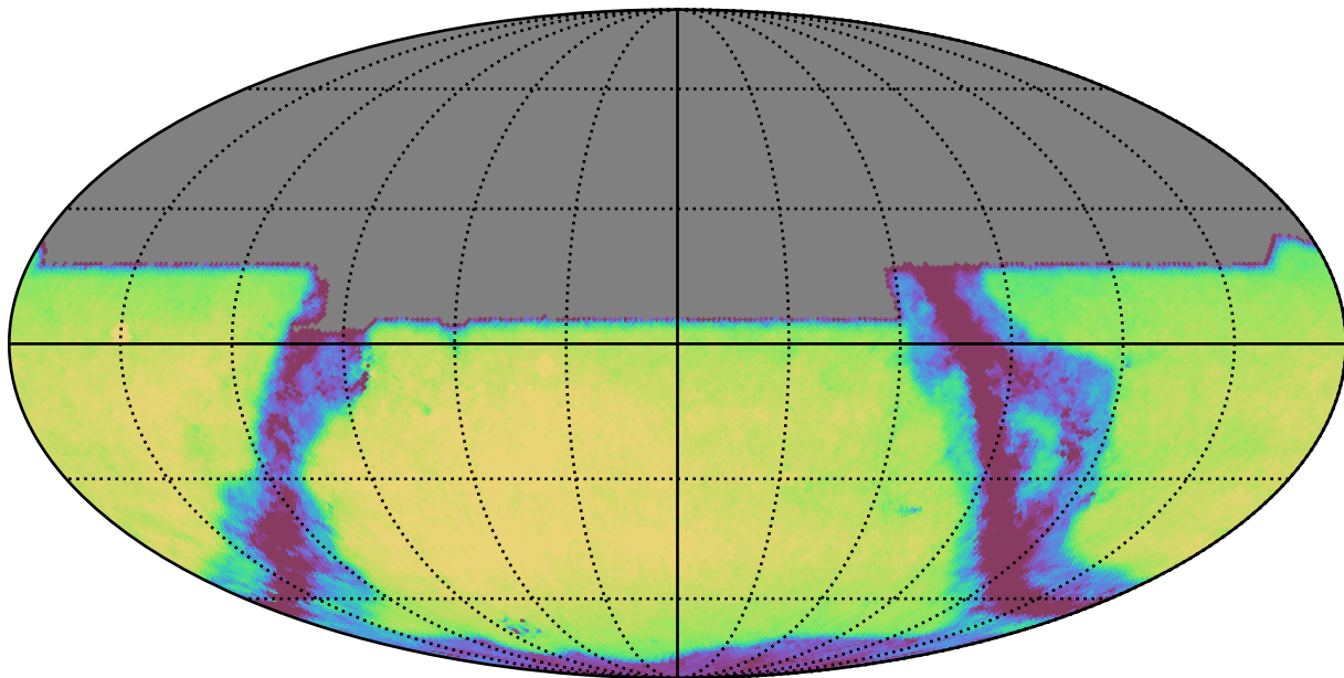
too_100_1v3.4_10yrs All sky y band: Exgal_CoaddM5
