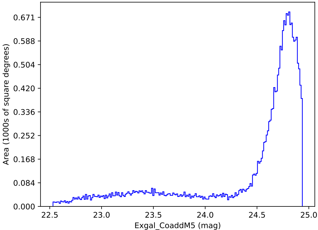
too_100_1v3.4_10yrs All sky y band: Exgal_CoaddM5
