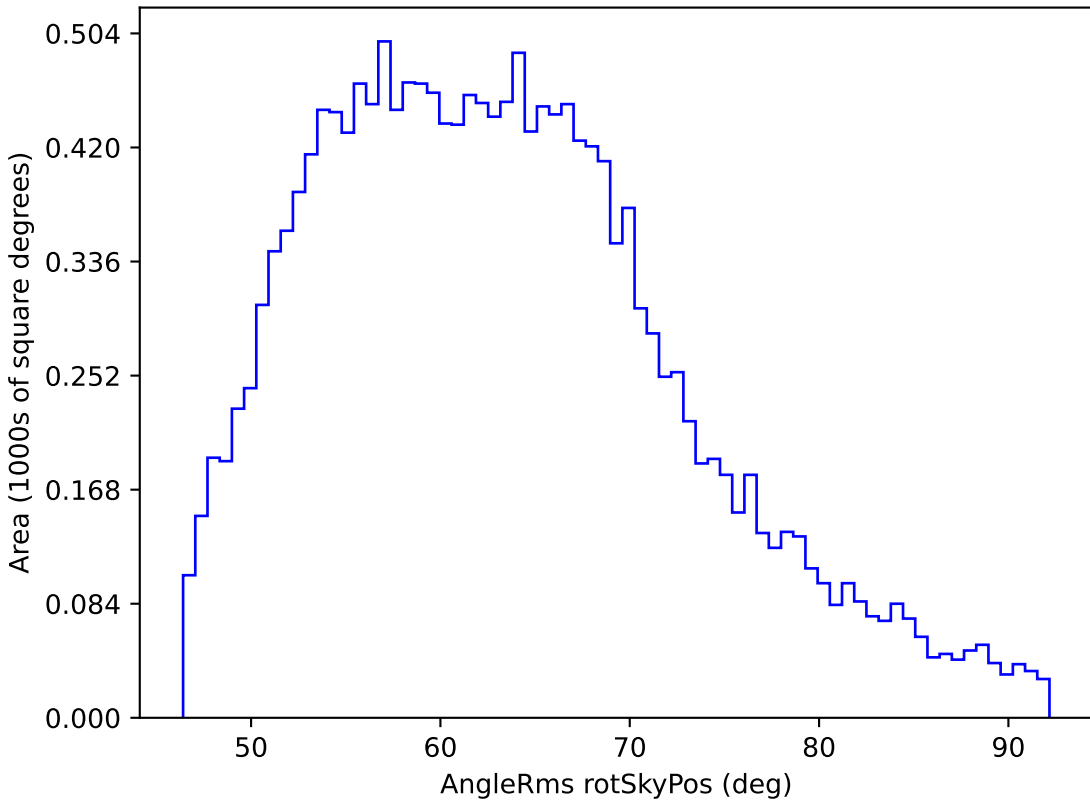
too_100_1v3.4_10yrs WFD y band: AngleRms rotSkyPos
