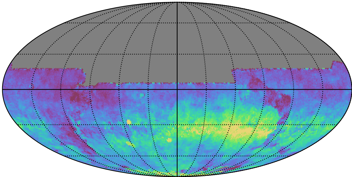
too_100_1v3.4_10yrs All sky y band: AngleRms rotSkyPos
