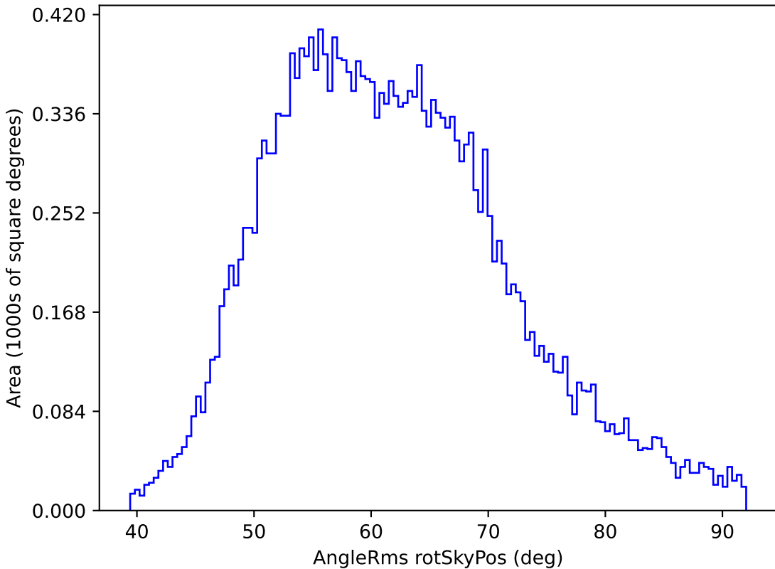
too_100_1v3.4_10yrs All sky y band: AngleRms rotSkyPos
