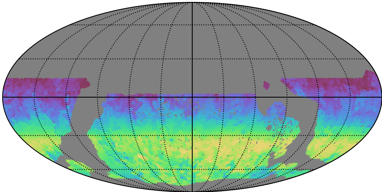
too_100_1v3.4_10yrs WFD z band: AngleRange rotSkyPos
