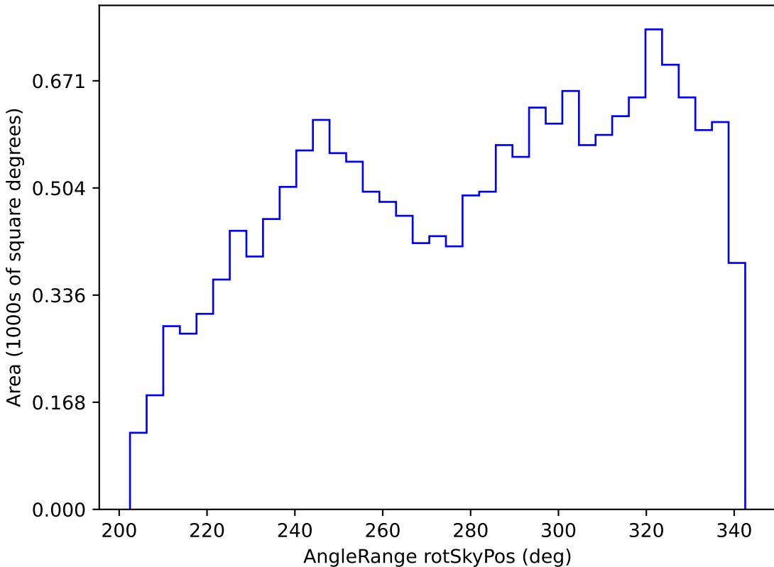
too_100_1v3.4_10yrs WFD z band: AngleRange rotSkyPos
