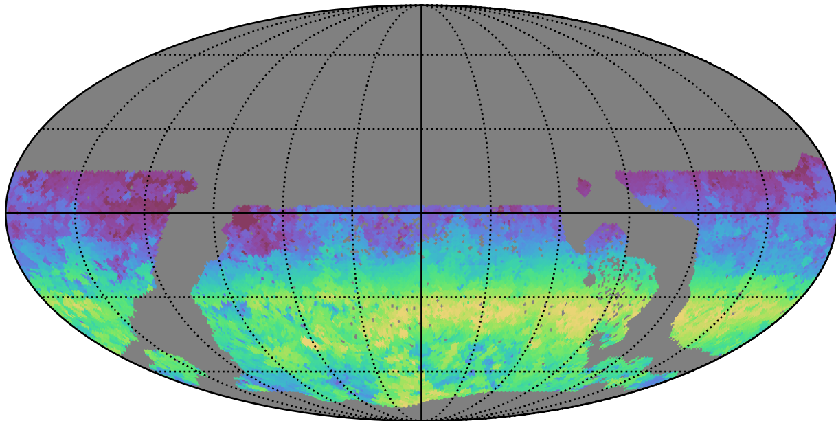
too_100_1v3.4_10yrs WFD y band: AngleRange rotSkyPos
