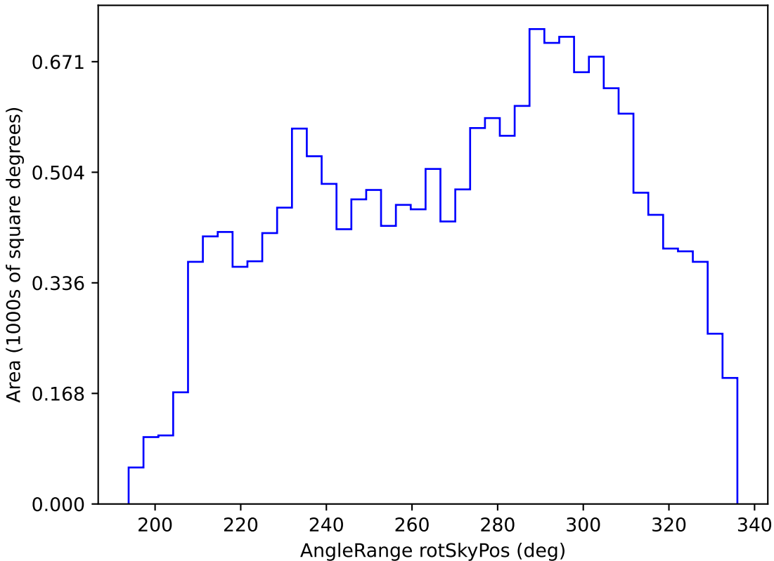
too_100_1v3.4_10yrs WFD y band: AngleRange rotSkyPos
