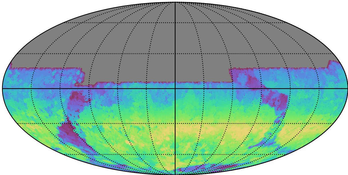
too_100_1v3.4_10yrs All sky y band: AngleRange rotSkyPos
