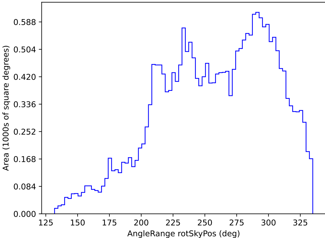
too_100_1v3.4_10yrs All sky y band: AngleRange rotSkyPos
