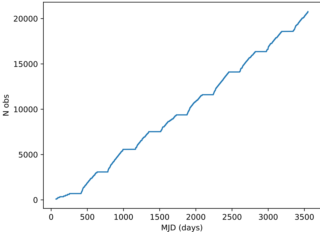
too_100_1v3.4_10yrs note like DD:ELAISS1%: Cumulative
