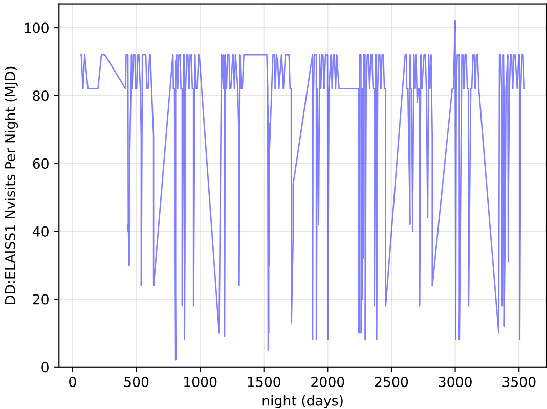
too_100_1v3.4_10yrs all bands: DD:ELAISS1 Nvisits Per Night
