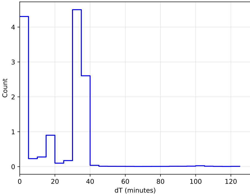
1e6 telescope_jerk_v3.5_10yrs All sky: DeltaT Histogram
