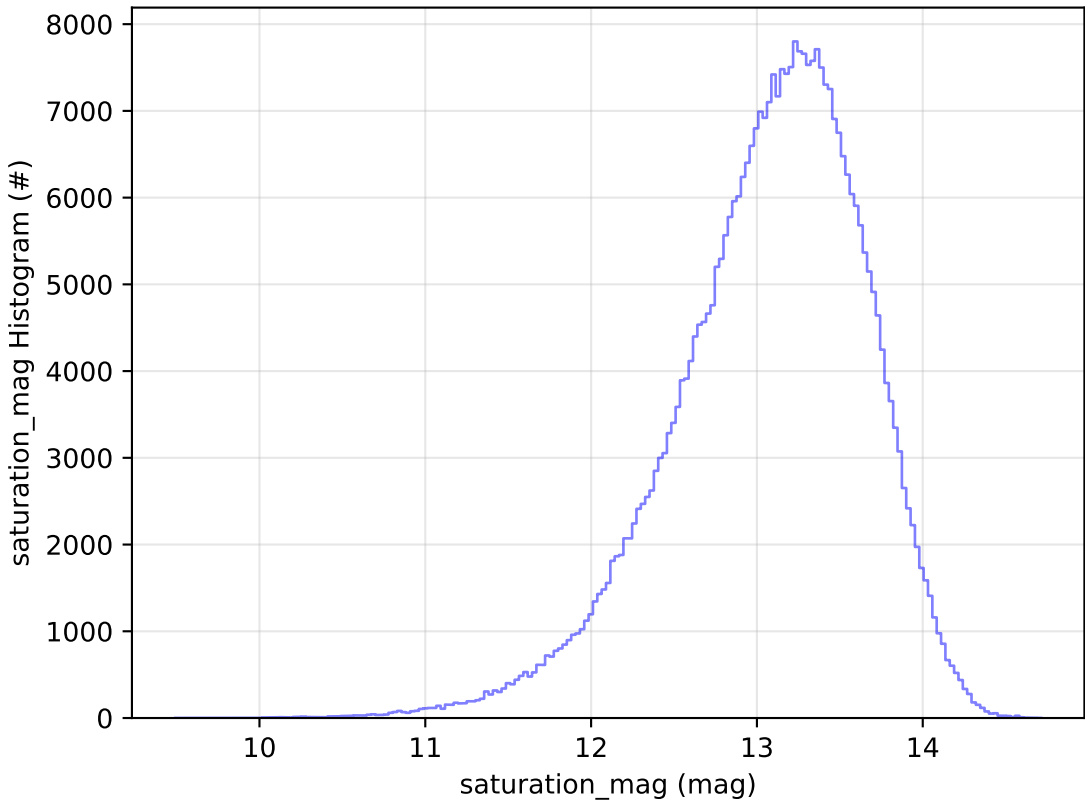
start_date_do90v3.4_10yrs WFD y band: saturation_mag Histogram
