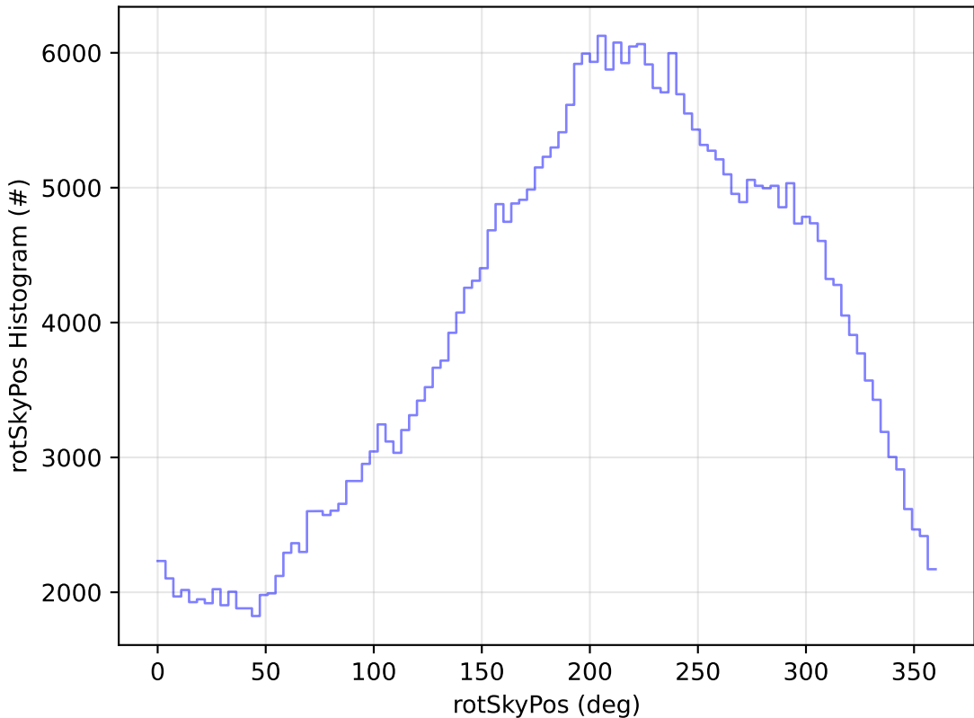
start_date_do90v3.4_10yrs WFD y band: rotSkyPos Histogram
