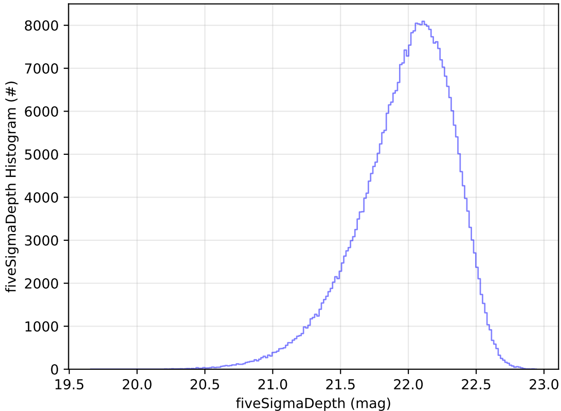
start_date_do90v3.4_10yrs WFD y band: fiveSigmaDepth Histogram
