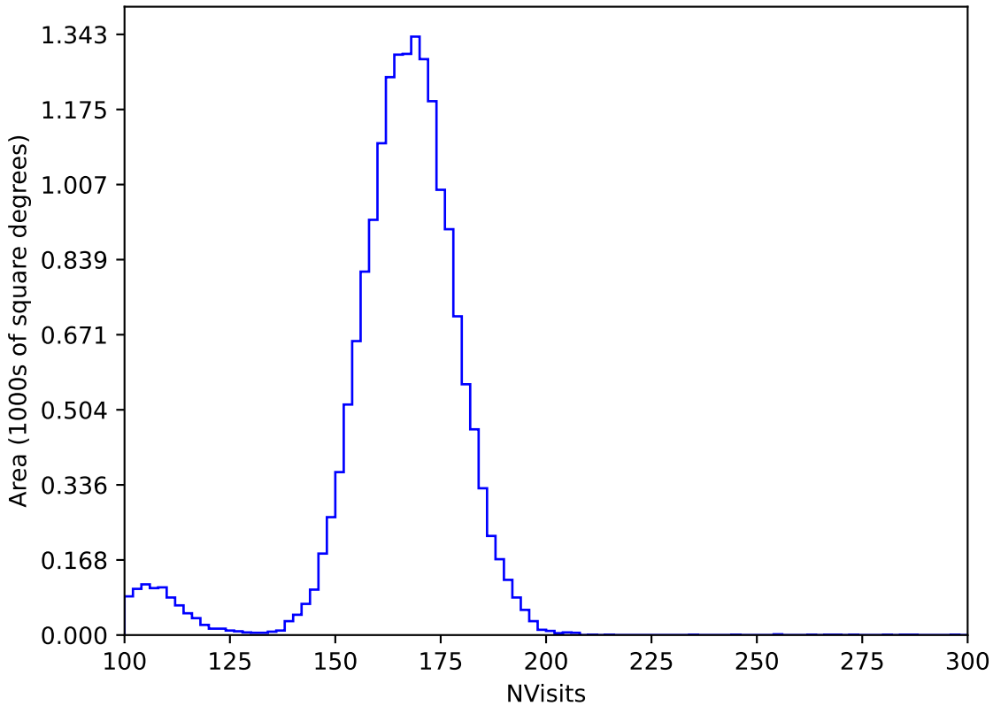
start_date_do90v3.4_10yrs WFD y band: NVisits
