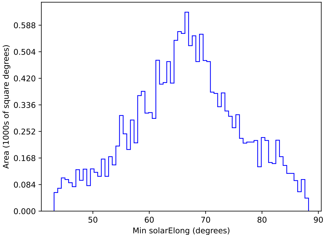
start_date_do90v3.4_10yrs WFD y band: Min solarElong
