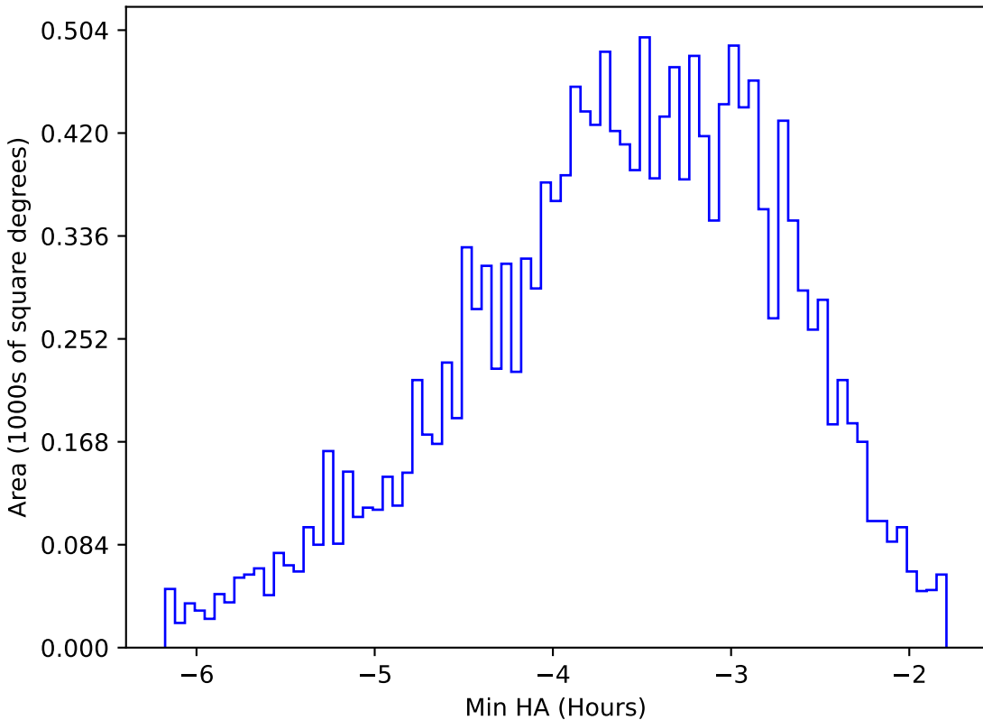
start_date_do90v3.4_10yrs WFD y band: Min HA
