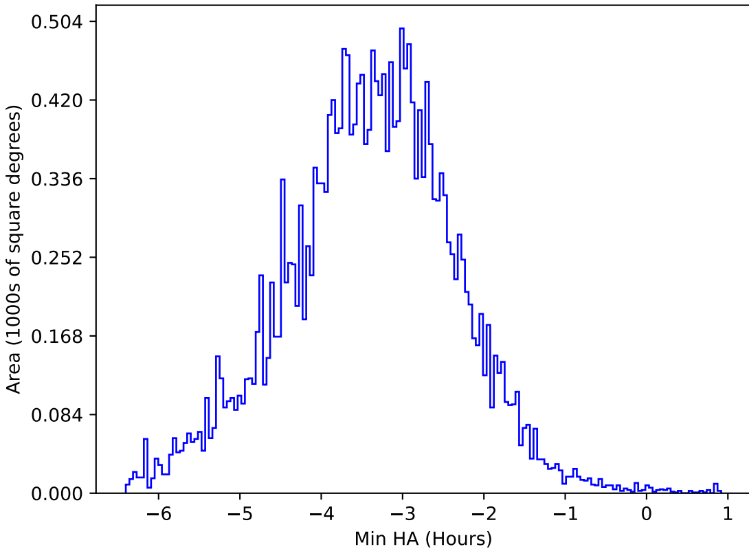
start_date_do90v3.4_10yrs All sky y band: Min HA
