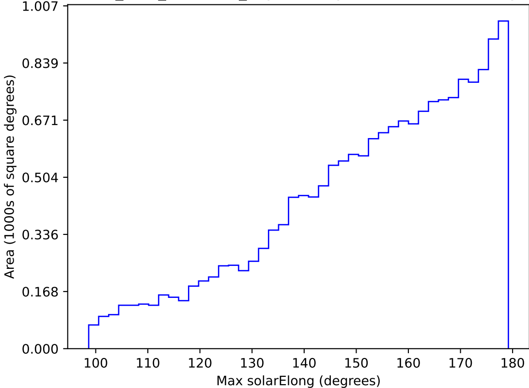
start_date_do90v3.4_10yrs WFD y band: Max solarElong
