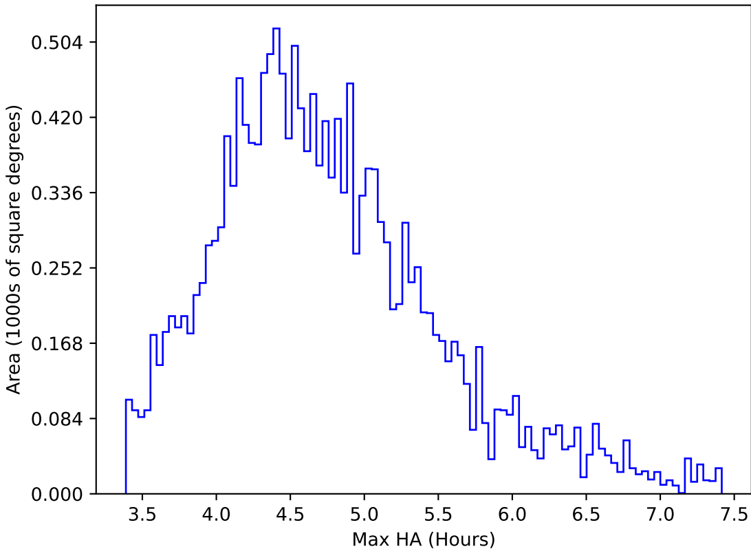
start_date_do90v3.4_10yrs WFD y band: Max HA
