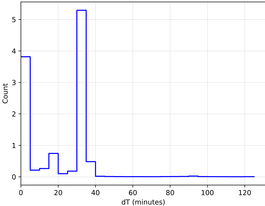
1e6 start_date_do90v3.4_10yrs WFD: DeltaT Histogram
