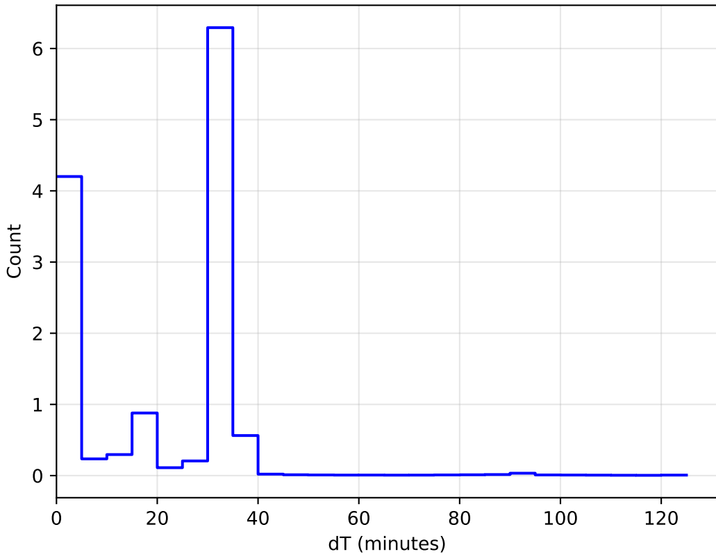
1e6start_date_do90v3.4_10yrs All sky: DeltaT Histogram
