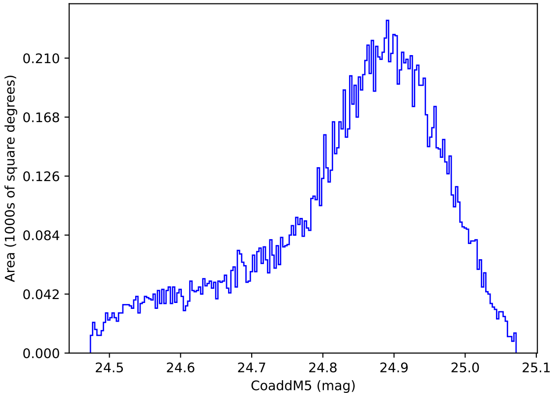
start_date_do90v3.4_10yrs WFD y band: CoaddM5
