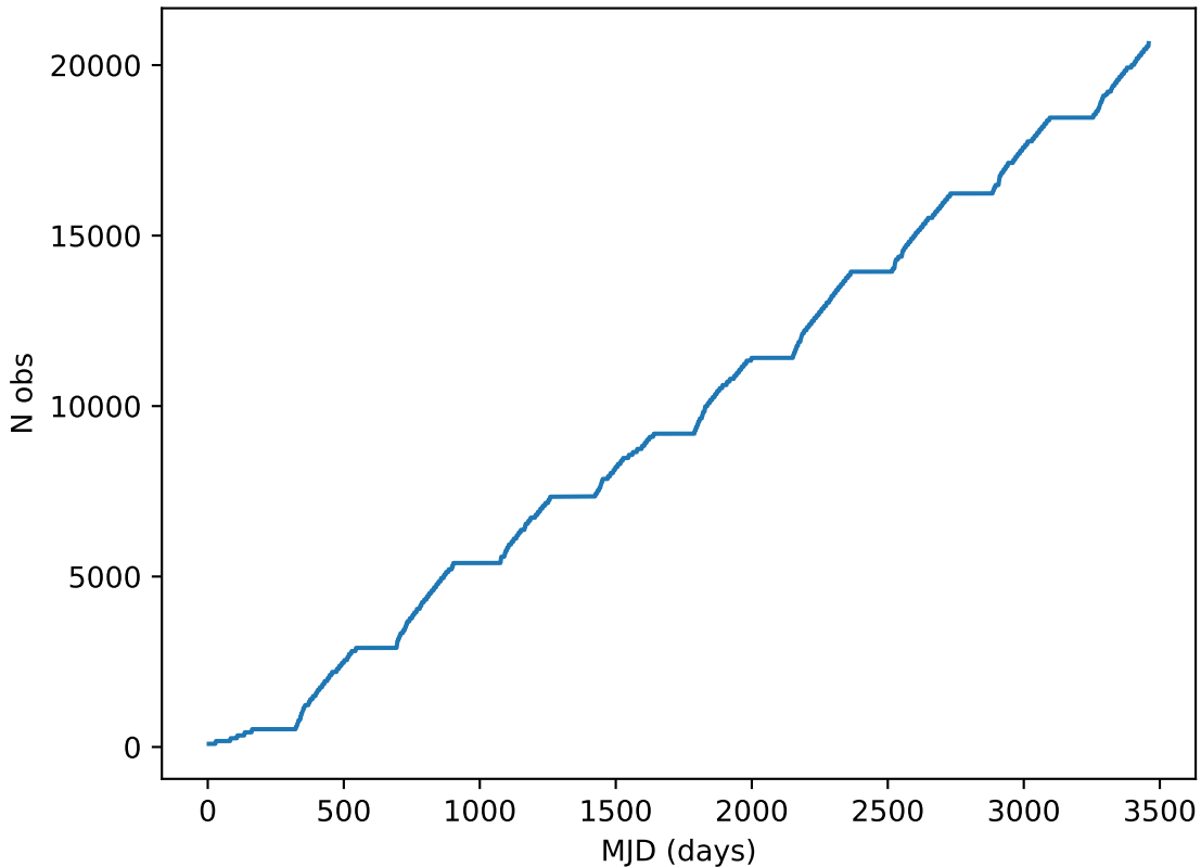
start_date_do90v3.4_10yrs all bands: DD:ELAISS1 Cumulative NVisits
