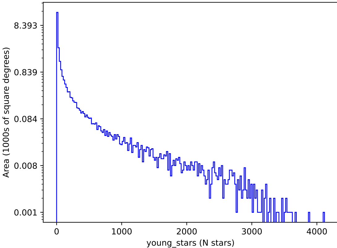
start_date_do360v3.4_10yrs : young_stars
