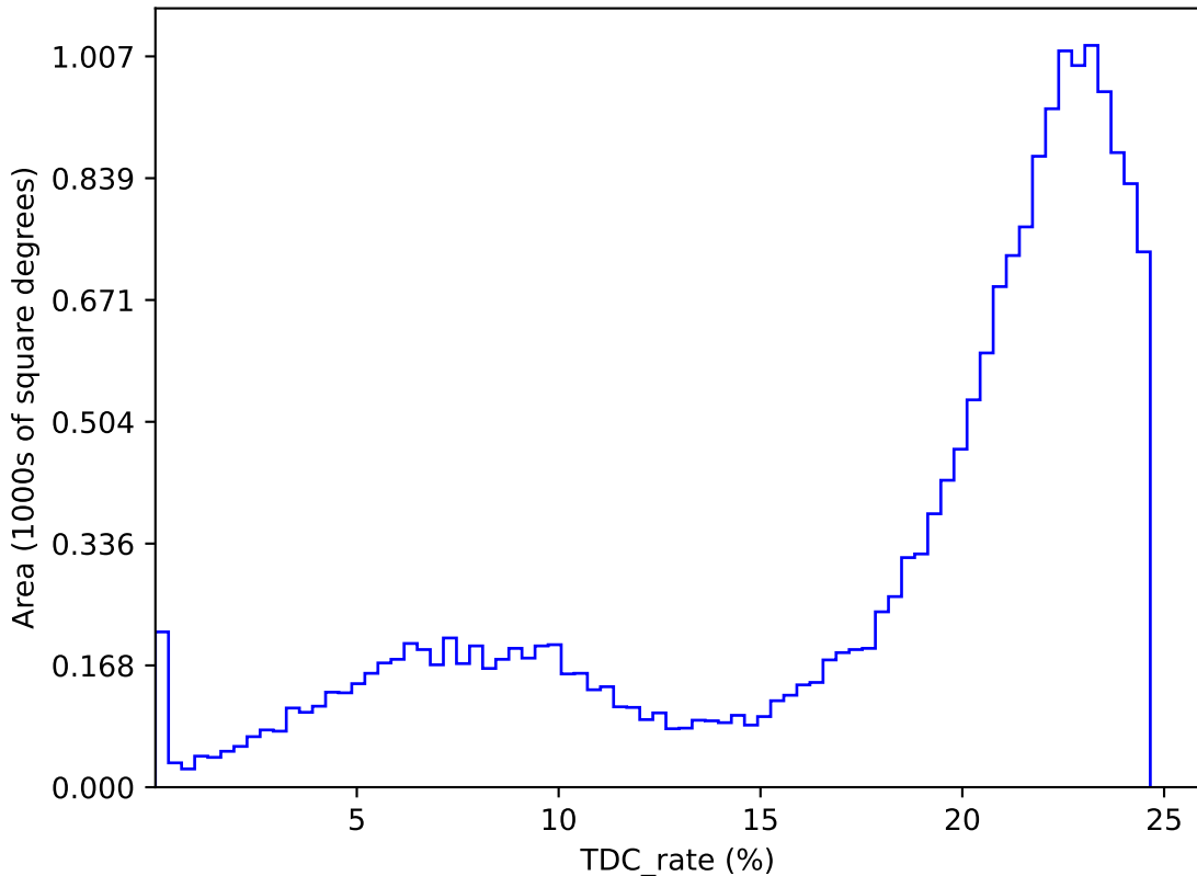
start_date_do360v3.4_10yrs : TDC_rate
