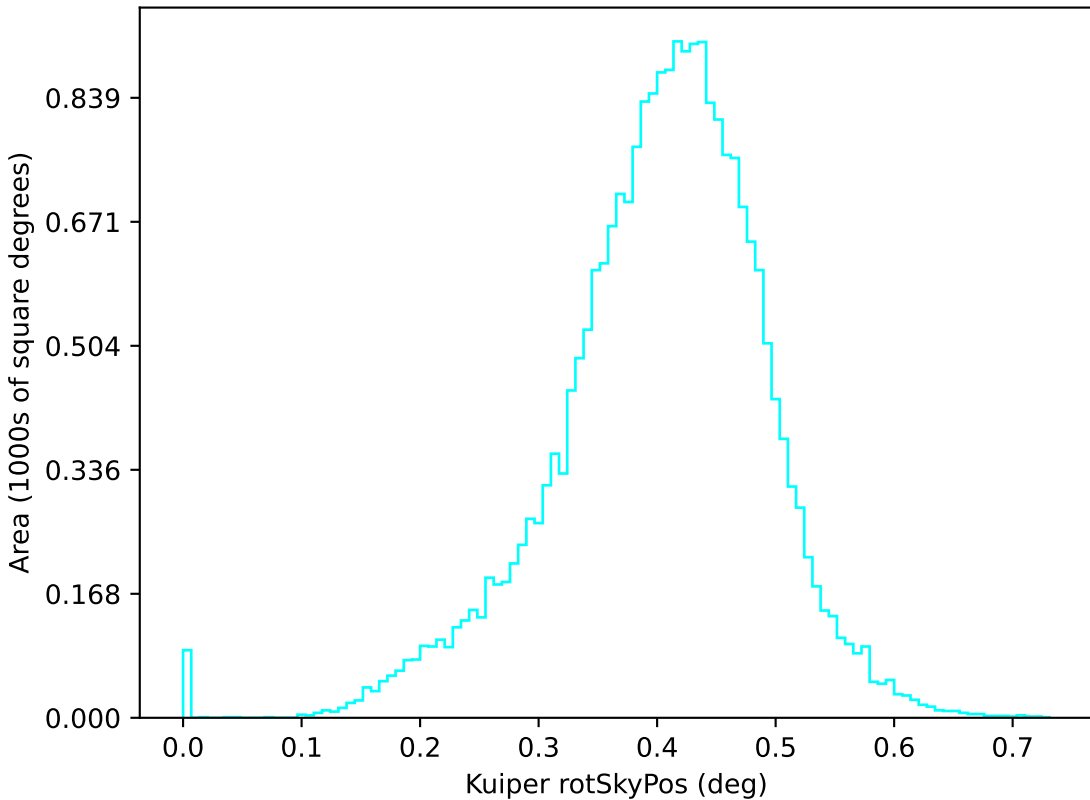
start_date_do360v3.4_10yrs u: Kuiper rotSkyPos
