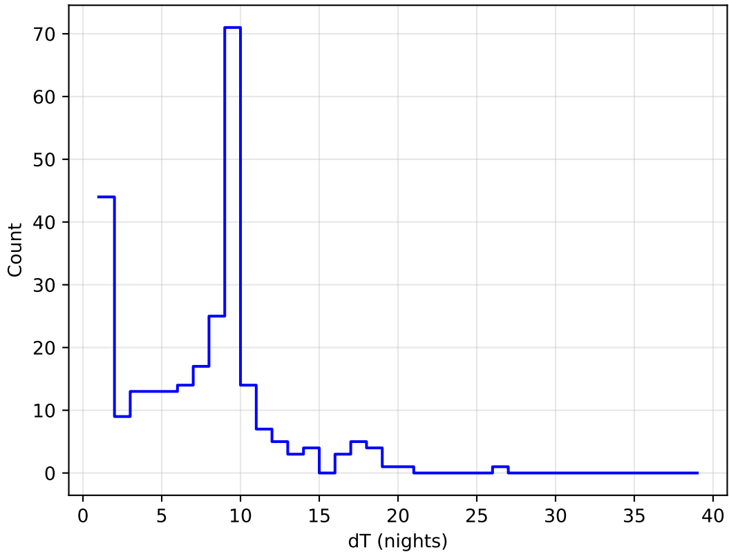
start_date_do360v3.4_10yrs all bands: DD:ELAISS1 Delta Nights Histogram
