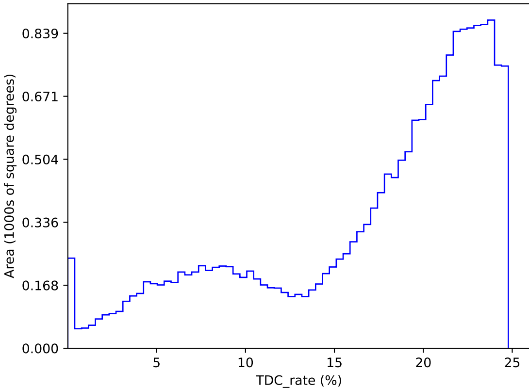
start_date_do270v3.4_10yrs : TDC_rate
